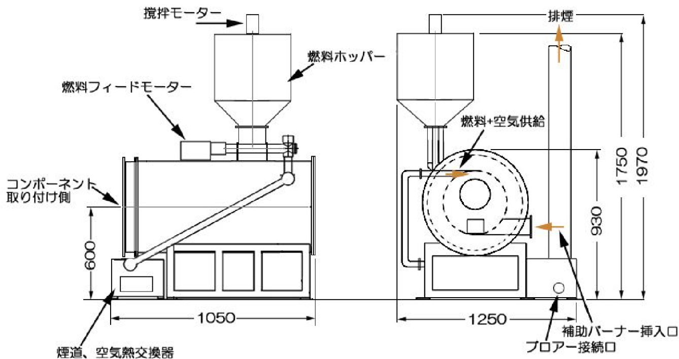
図一 4 燃焼炉の外形寸法
